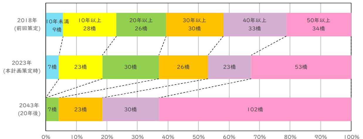
図.架設経過年数の割合
