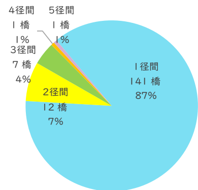
図. 径間数毎の割合
