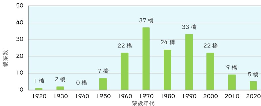
図.年代別架設橋梁数
