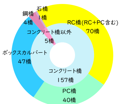
図. 橋梁形式毎の割合
