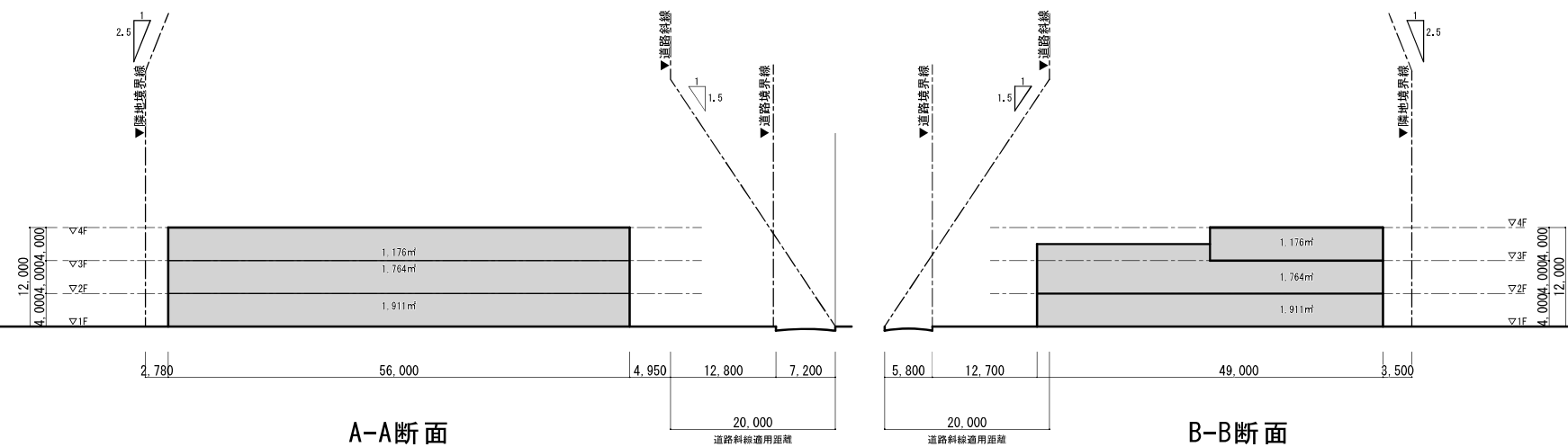
断面図 S=1/800
